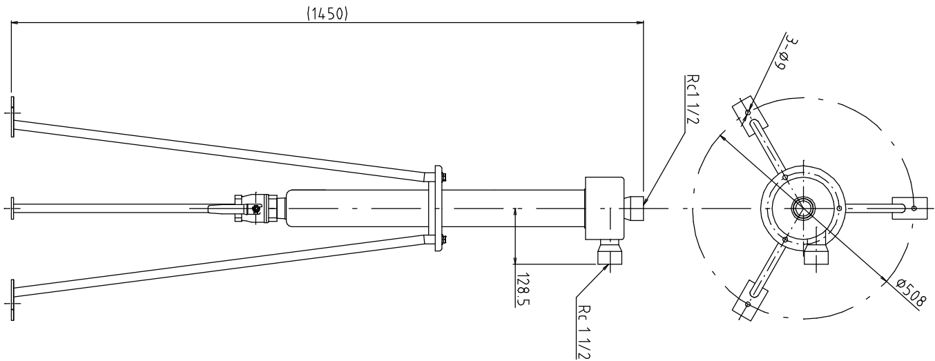
【フアンカー取付図】
