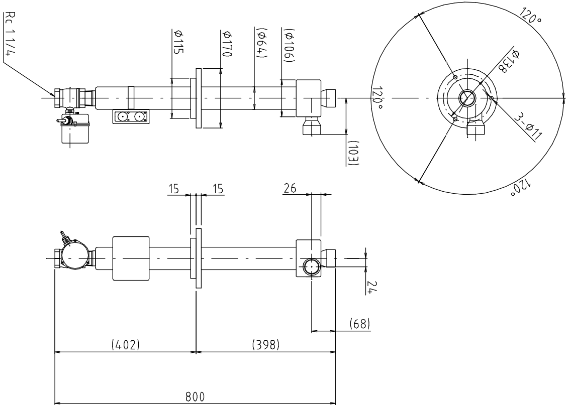
【フィルスター本体（三脚無し）詳細】
