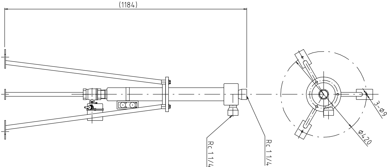
【フソカ〜取付図】
