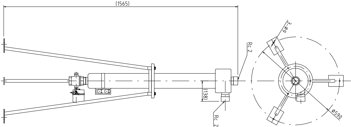
【ファンカー取付図】
