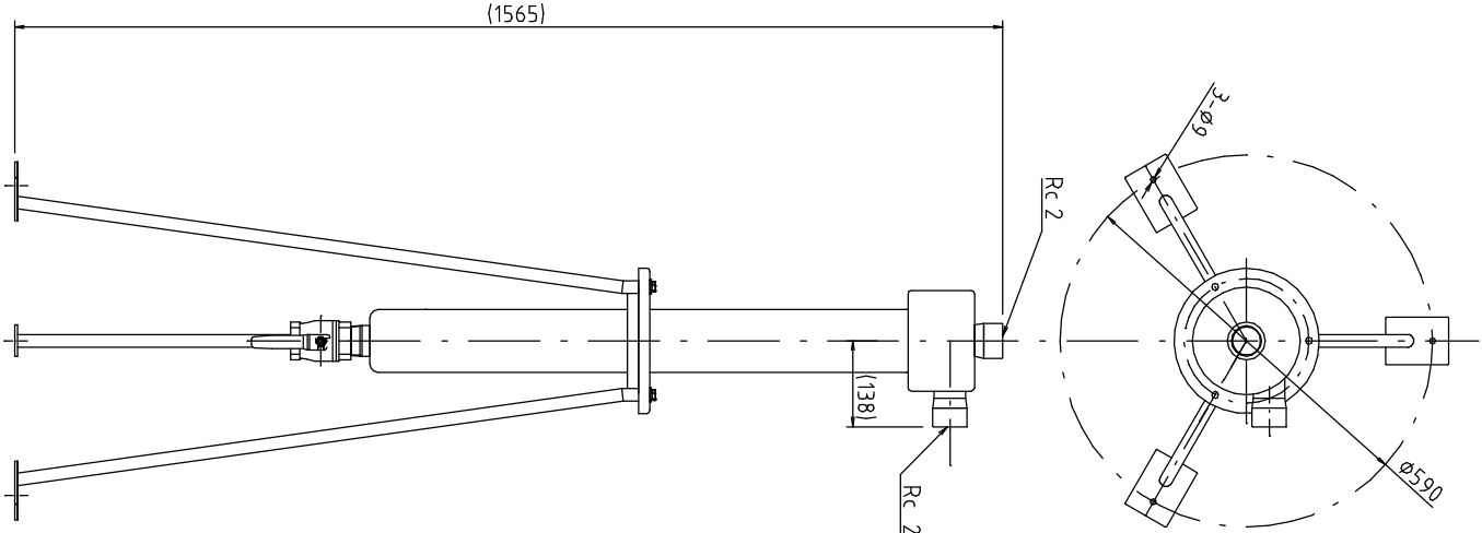
【フソカー取付図】
